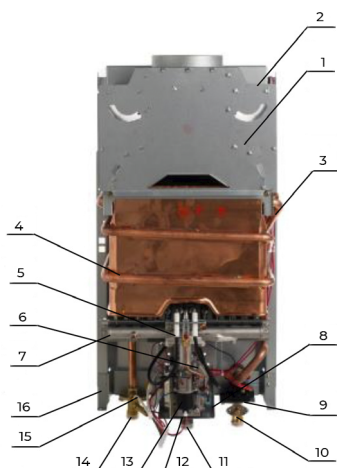
Рис. 1б. Аппарат водонагревательный проточный газовый бытового MIZUDO (модель с электронной модуляцией пламени)
