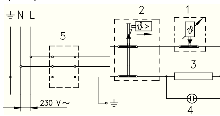
Электросхема
