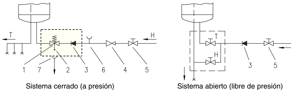
Sistema cerrado (a presión)
