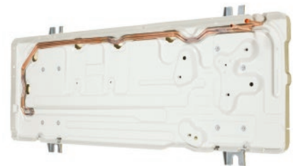
Трубка хладагента проложена по днищу наружного блока
