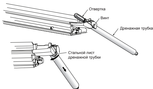
Дренажная трубка
