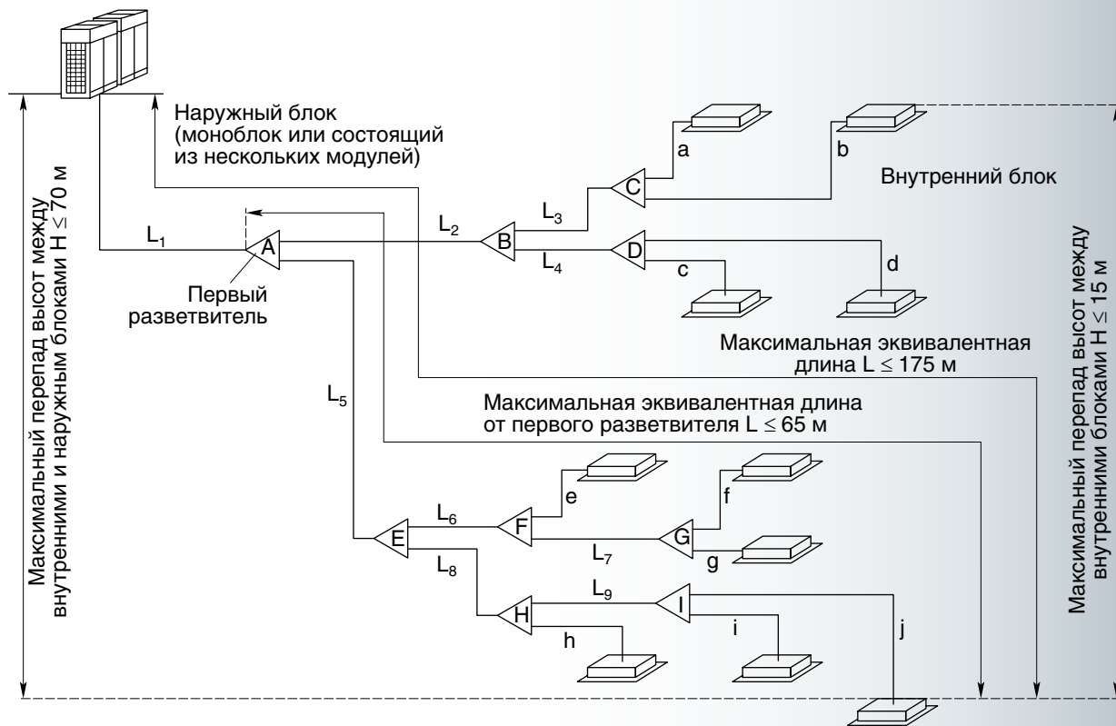
Рис. 1. Система трубопроводов мультизональной системы кондиционирования CMV-II
