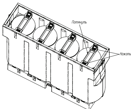
Рисунок 22. Снятие прижима HEPA-фильтра
