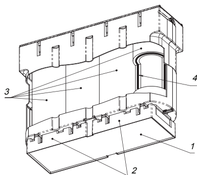
Рисунок 2. Устройство фильтрующего модуля
