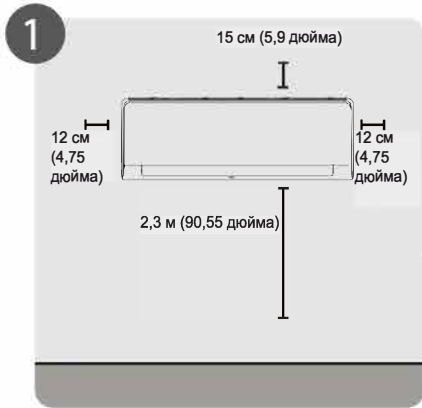
1 Выберите место установки
