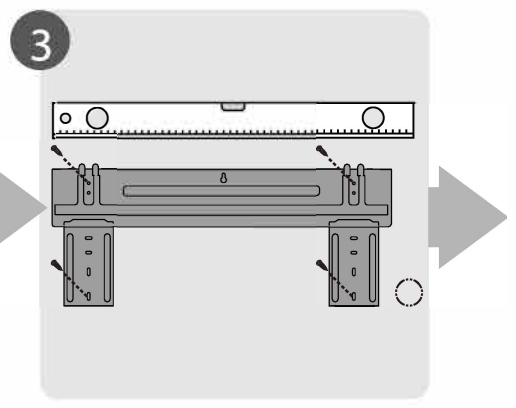
3 Закрепите монтажную пластину
