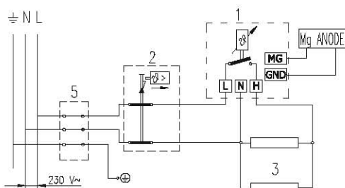
Elektriskā shēma
